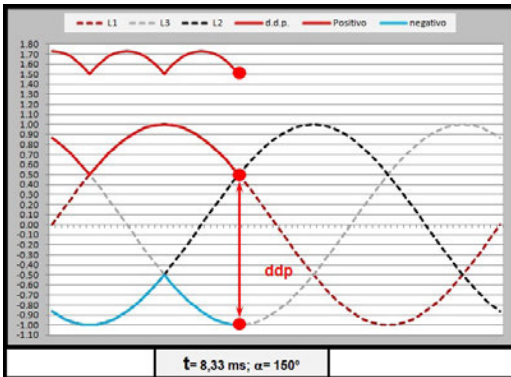
Figura 9 – Valor de tensión continua en el instante t = 8,83 ms
