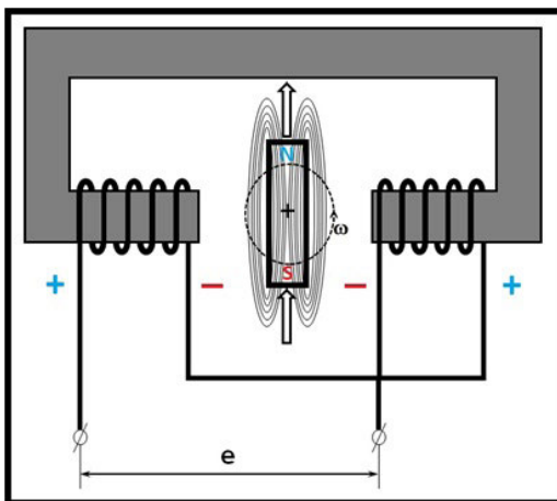
Figura 1- Generador monofásico
