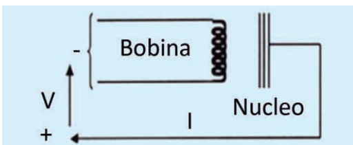
Figura 2. Prueba de Aislamiento en cc
