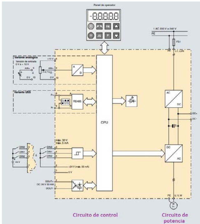
Figura 1- Esquema de bloques de un variador de frecuencias.
