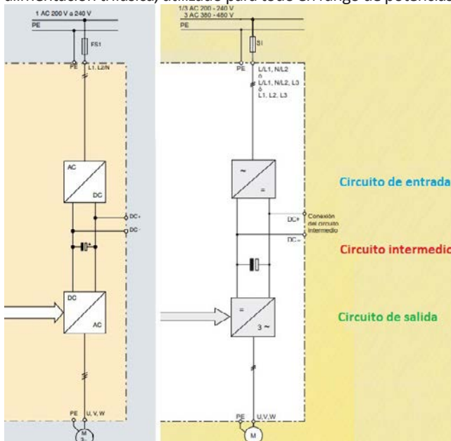
Figura 2- Esquema de potencia de un variador de frecuencias.
