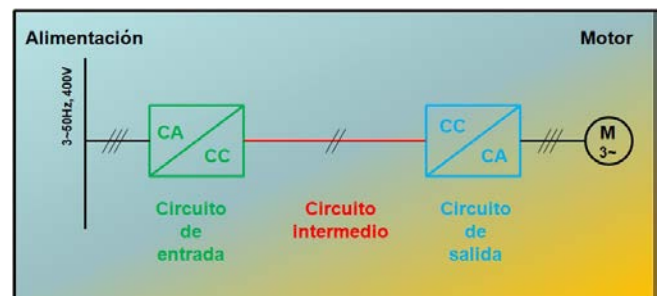
Figura 3- Circuito de potencia de un variador de frecuencias.
